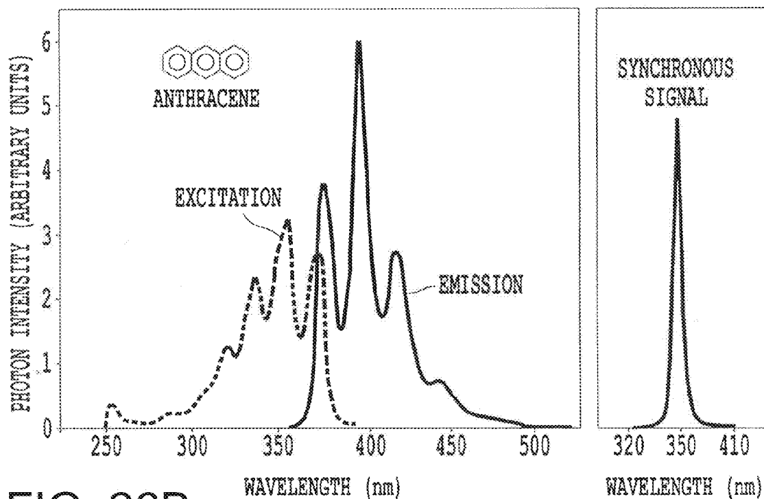
FIG. 26B
