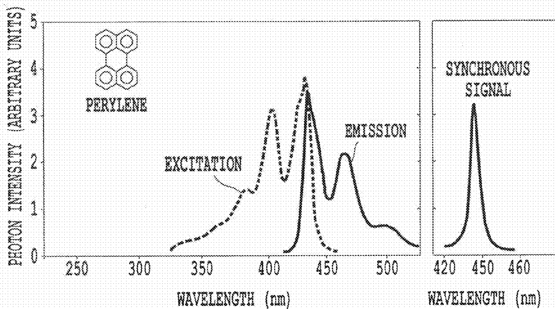
FIG. 26C
