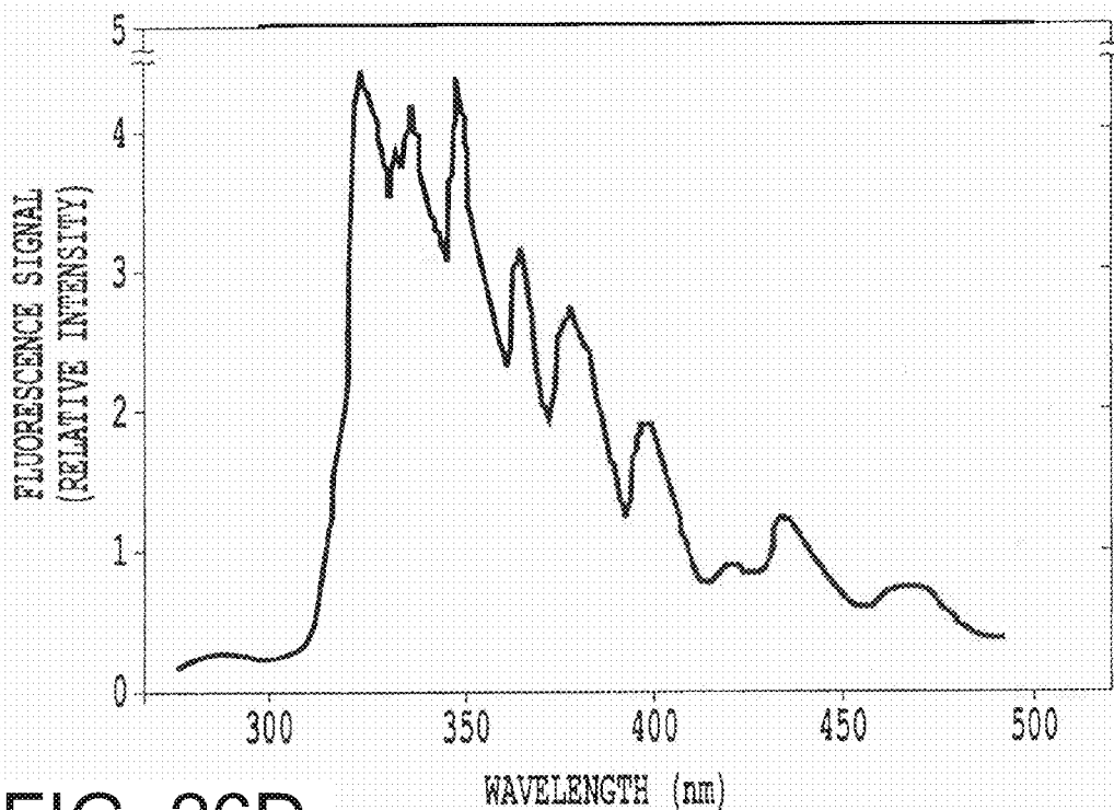
FIG. 26D
